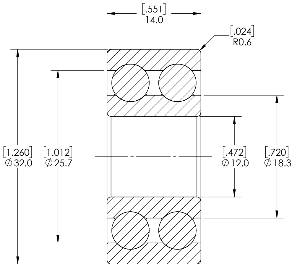
SECTION A-A
