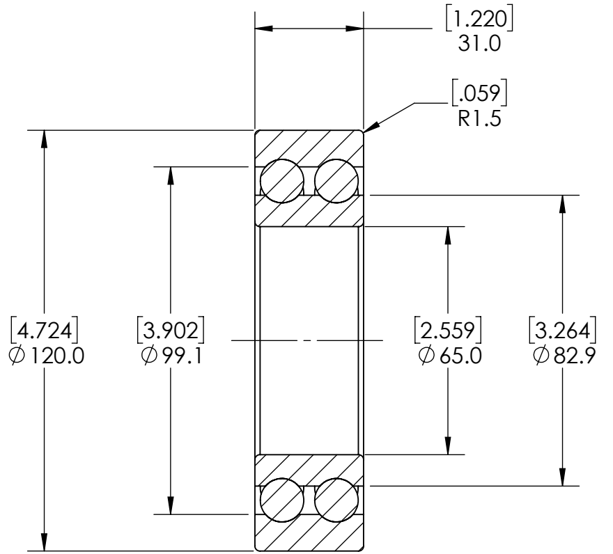
SECTION A-A
