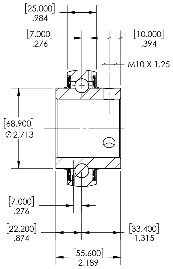
SECTION A-A
