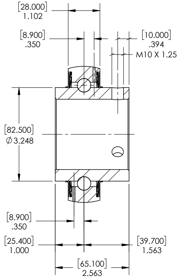
SECTION A-A
