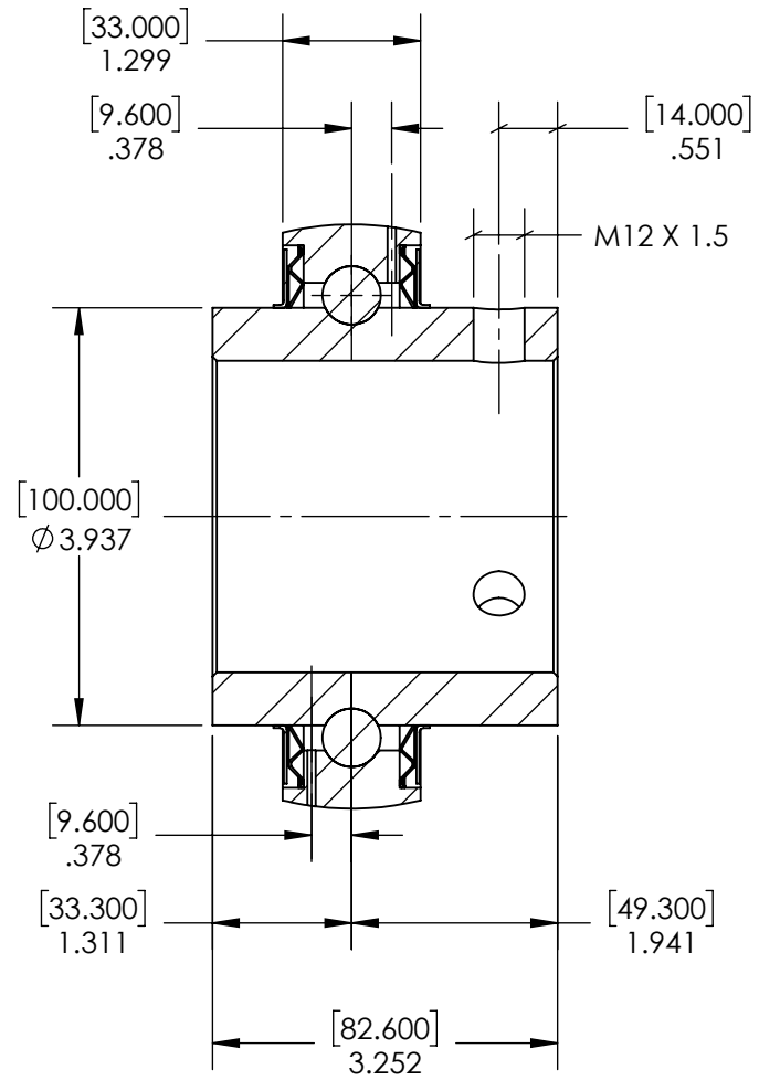
SECTION A-A
